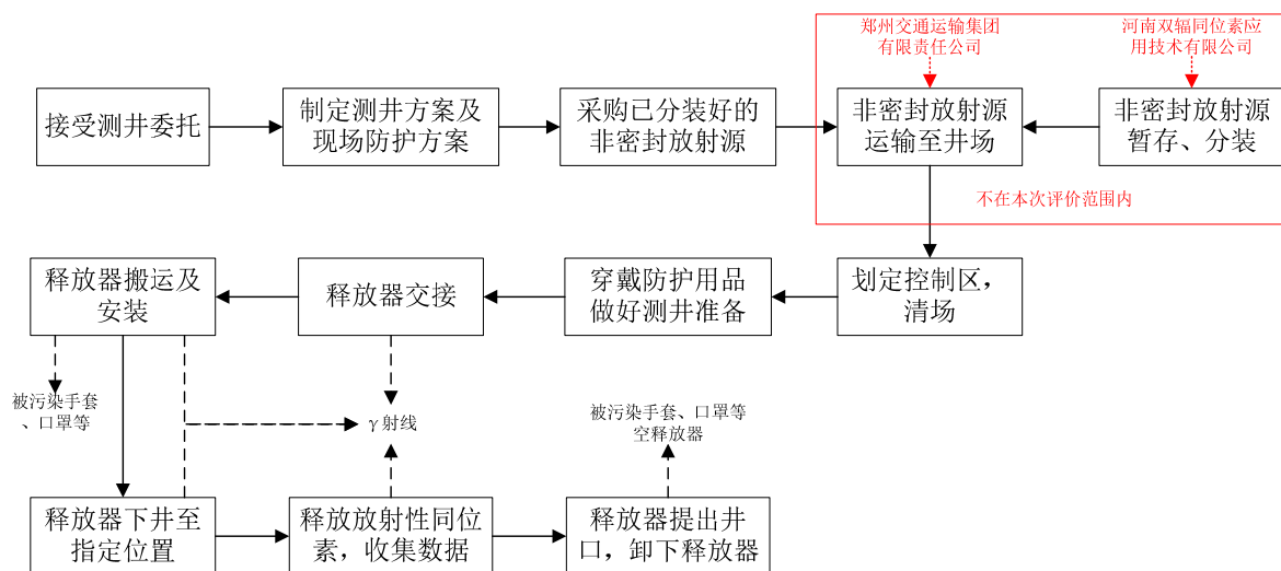
图 9-4 非密封放射源测井工艺流程及产排污环节示意图
